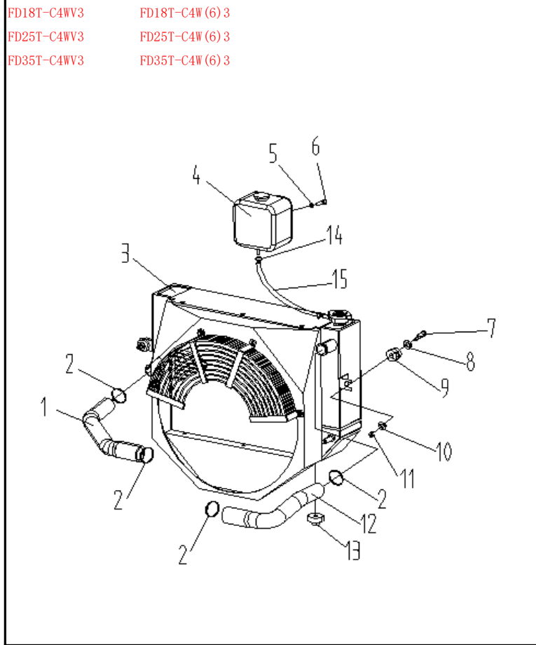
图5/Fig5. 散热器及安装/COOLING SYSTEM MOUNT
