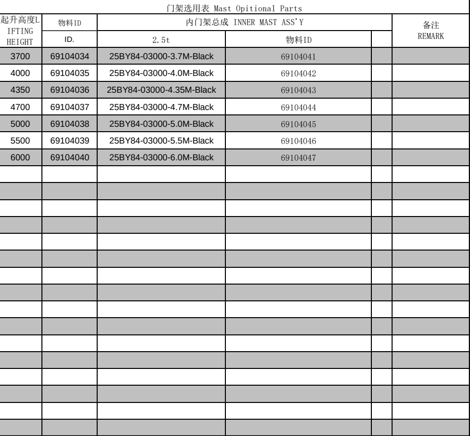
门架(三级全自由)/MAST(FULL FREE 3-STAGE MAST)
