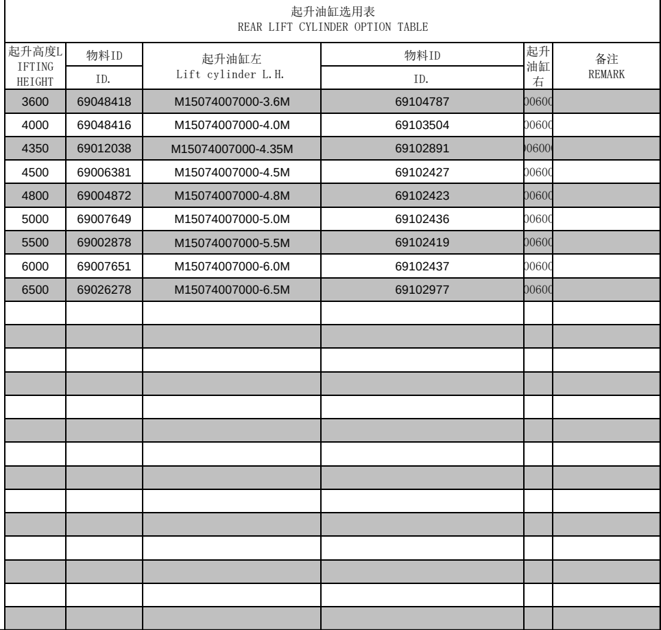
后起升油缸(三级全自由)/REAR LIFT CYLINDER(FULL FREE 3-STAGE MAST)
