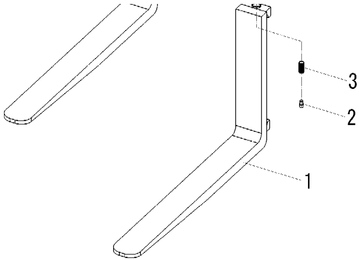
图55/Fig55. 货叉/FORK
