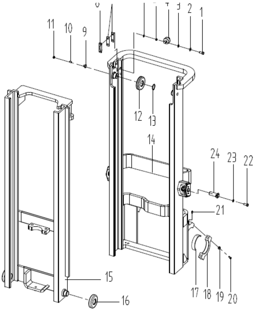
图51/FIG. 51 门架(三级全自由)/MAST(FULL FREE 3-STAGE MAST)
