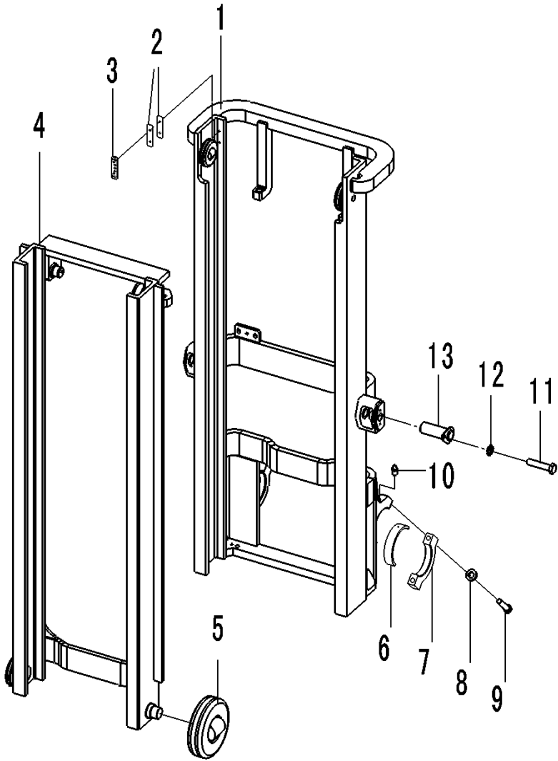
图46/FIG. 46 门架(基本型)/MAST(NORMAL MAST)
