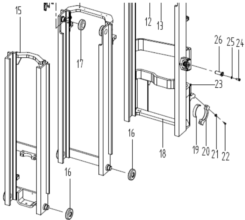
图51/FIG. 51 门架(三级全自由)/MAST(FULL FREE 3-STAGE MAST)
