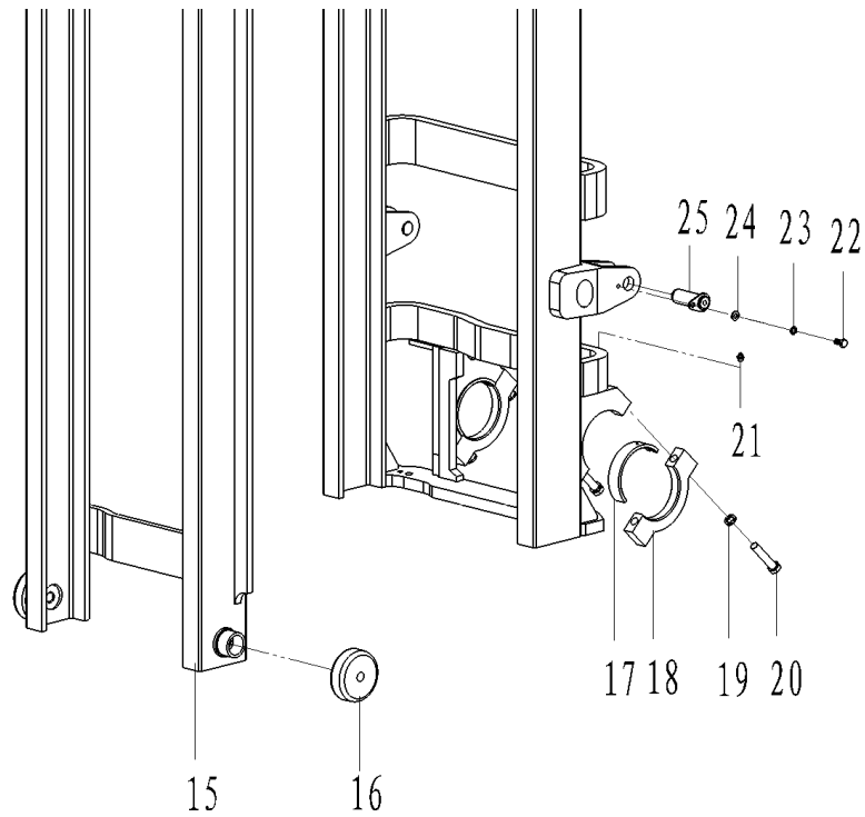
图43/FIG. 43 门架(基本型) / MAST (NORMAL MAST)
