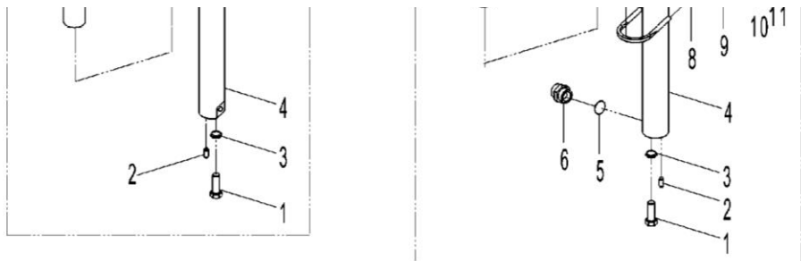
图52/FIG. 52 起升油缸(基本型)/LIFT CYLINDER(NORMAL MAST)
