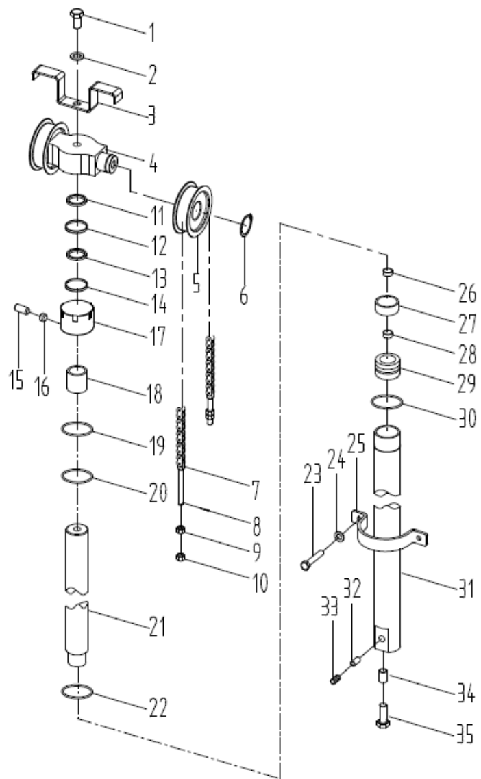
图58/FIG. 58 前起升油缸(二级全自由)/FRONT LIFT CYLINDER(FULL FREE 2-STAGE MAST)
