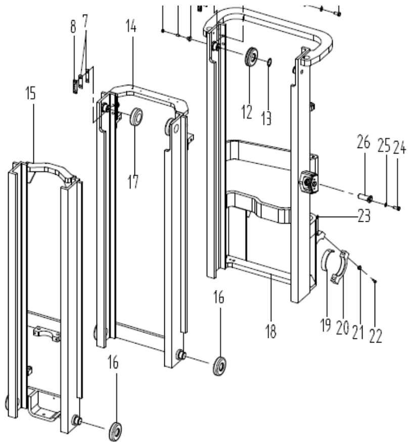
图51/FIG. 51 门架(三级全自由)/MAST(FULL FREE 3-STAGE MAST)
