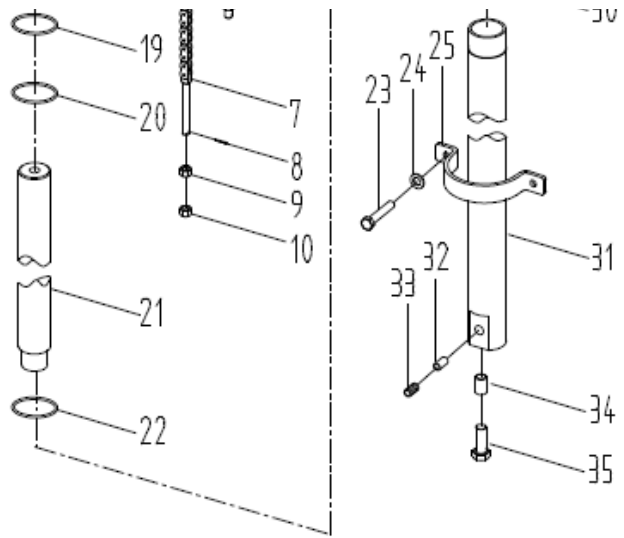
图61/Fig. 61 后起升油缸(三级全自由)/REAR LIFT CYLINDER(FULL FREE 3-STAGE MAST)
