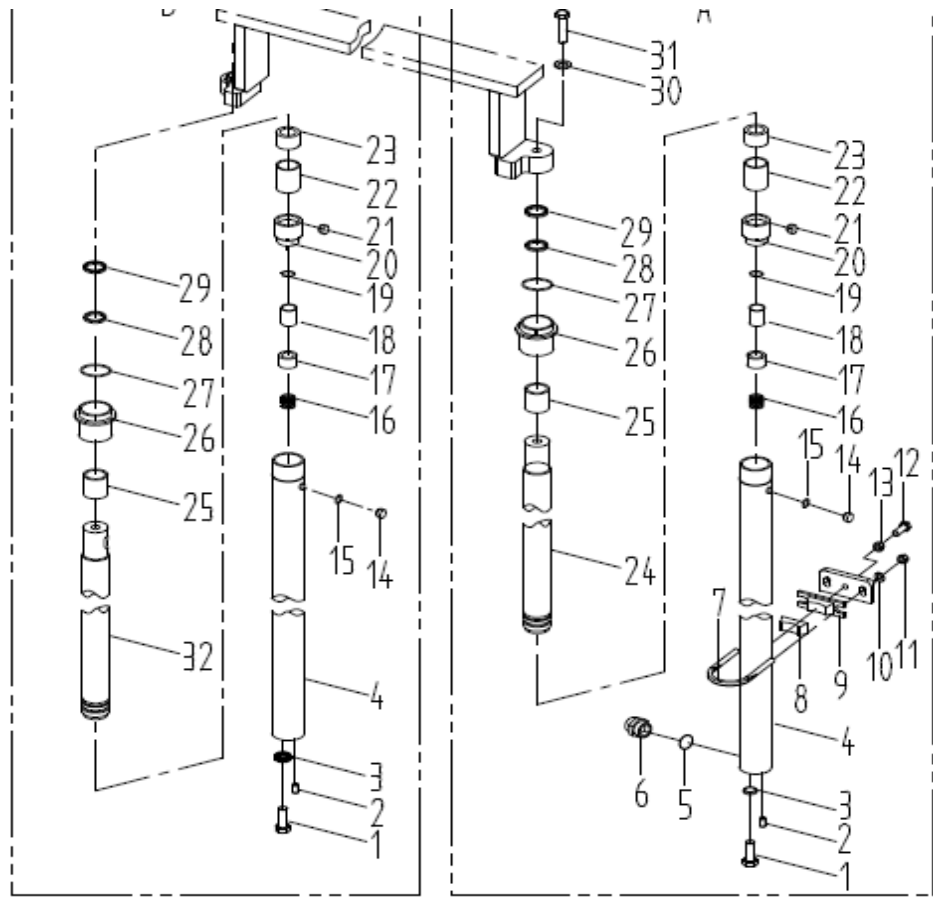
图59/FIG. 59. 后起升油缸(二级全自由)/REAR LIFT CYLINDER(FULL FREE 2-STAGE MAST)
