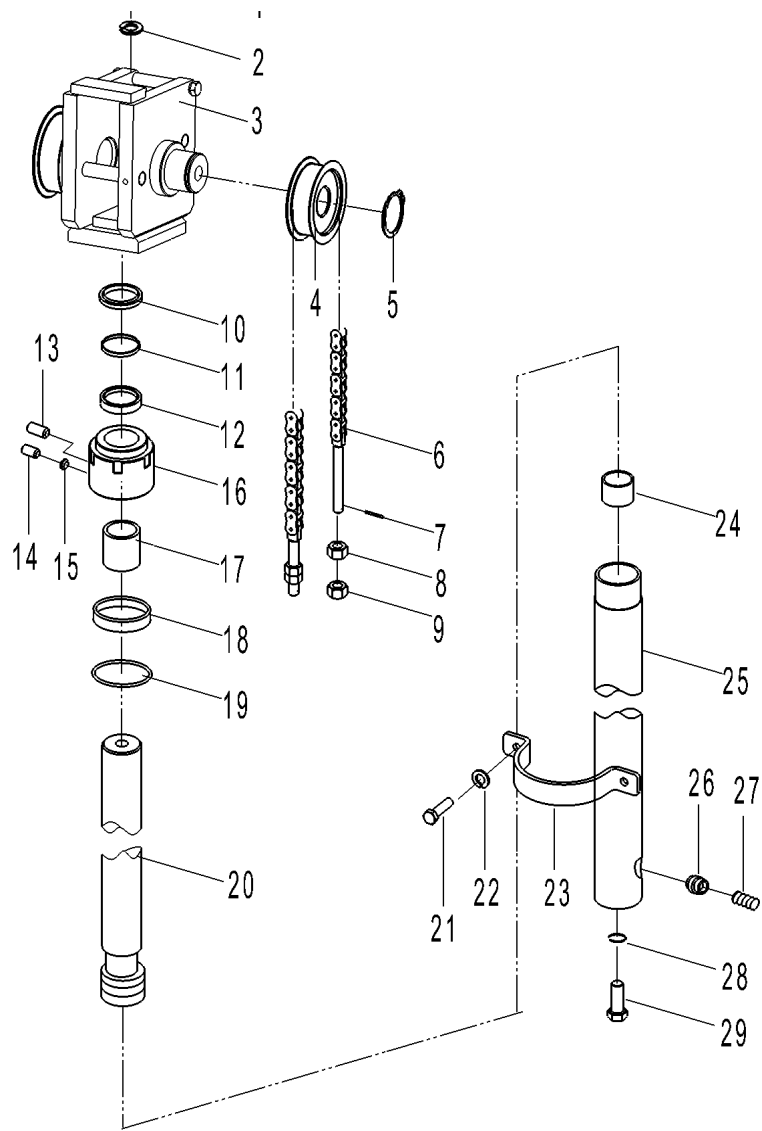
图54/FIG. 54 后起升油缸(二级全自由)/REAR LIFT CYLINDER(FULL FREE 2-STAGE MAST)
