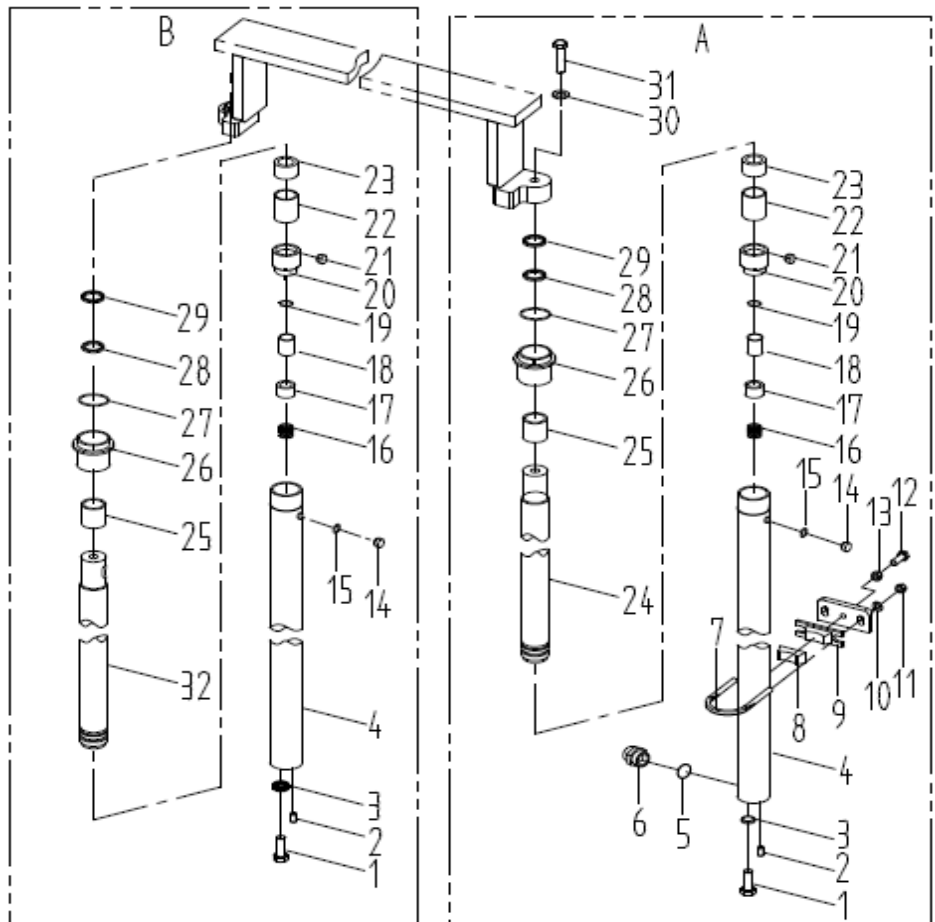
图59/FIG. 59. 后起升油缸(二级全自由)/REAR LIFT CYLINDER(FULL FREE 2-STAGE MAST)
