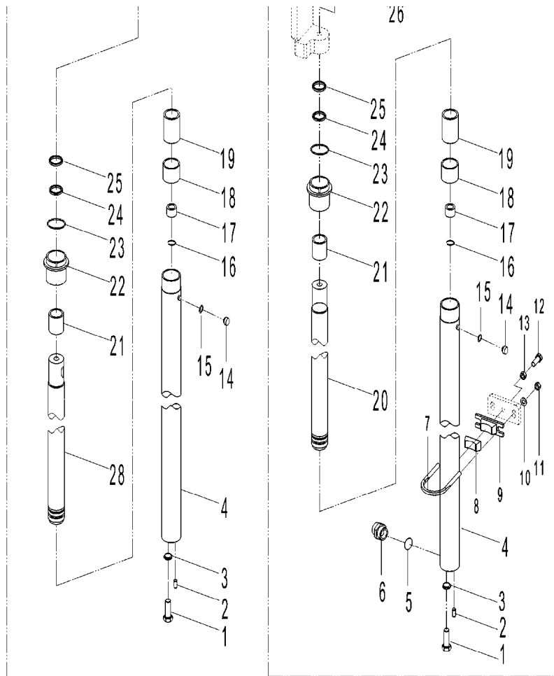
图55/FIG. 55 前起升油缸(三级全自由)/FRONT LIFT CYLINDER(FULL FREE 3-STAGE MAST)
