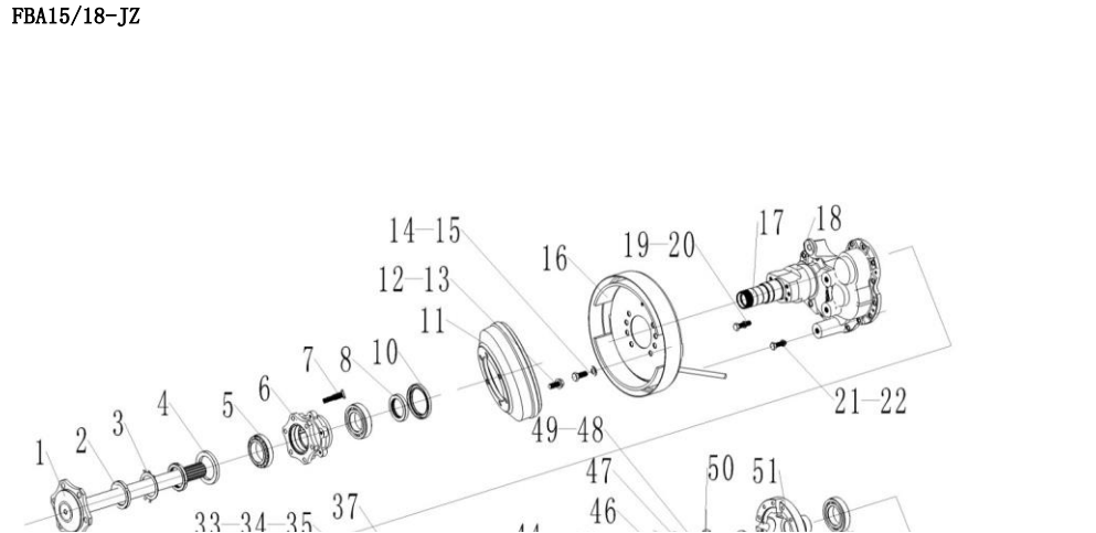
图3/Fig. 3 桥箱(华鹰HYMX1531000)/ DRIVE AXLE
