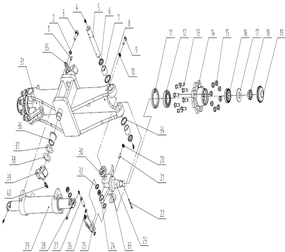
图19/Fig. 19 2. 5T转向桥(林德)/ STEERING AXLE
