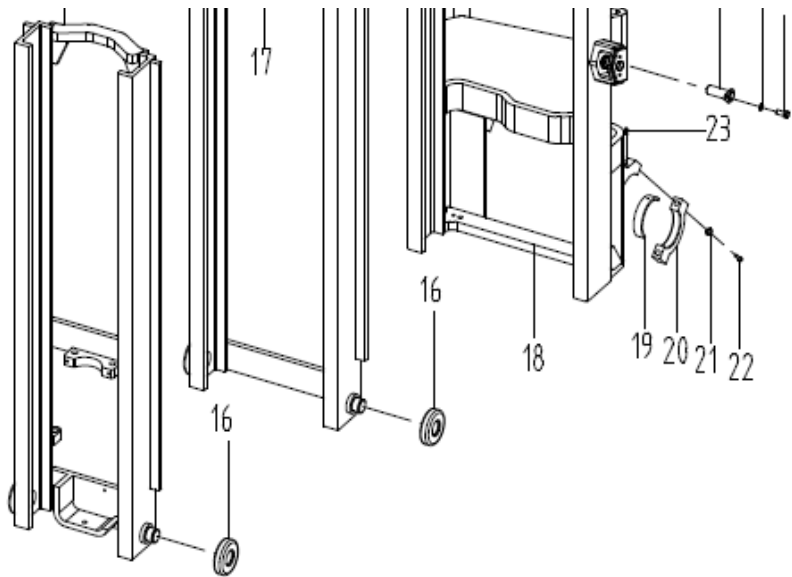
门架(三级全自由)/MAST(FULL FREE 3-STAGE MAST)
