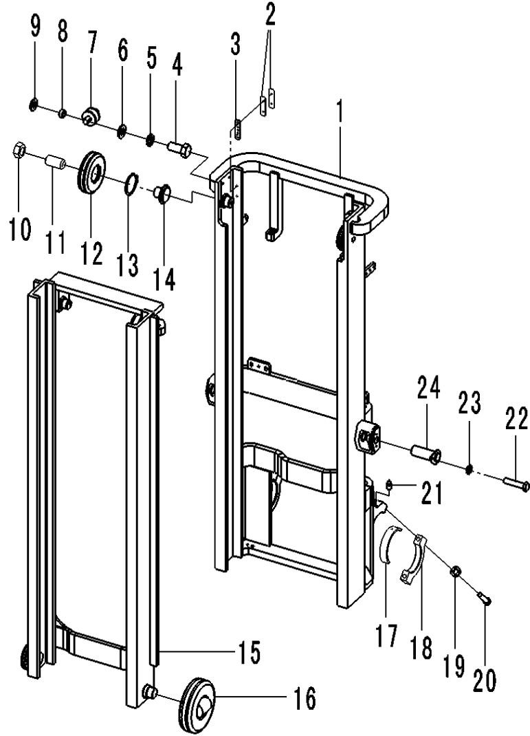
门架(二级全自由)/MAST(FULL FREE 2-STAGE MAST)
