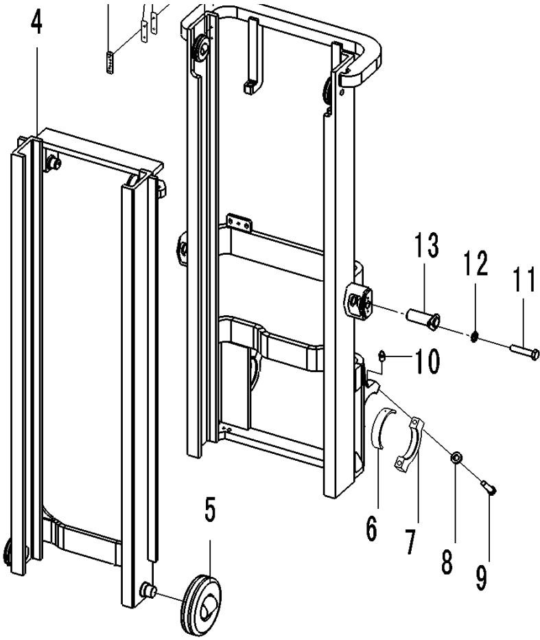
图47/FIG. 47 门架(二级全自由)/MAST(FULL FREE 2-STAGE MAST)
