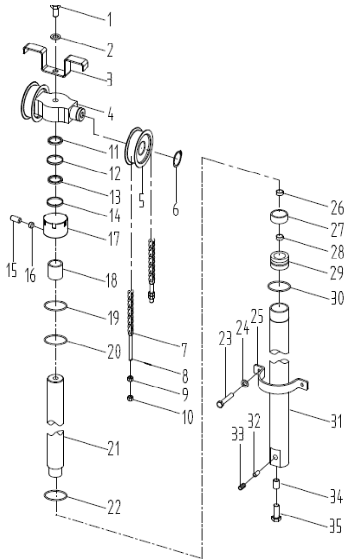
图59/FIG. 59. 后起升油缸(二级全自由)/REAR LIFT CYLINDER(FULL FREE 2-STAGE MAST)
