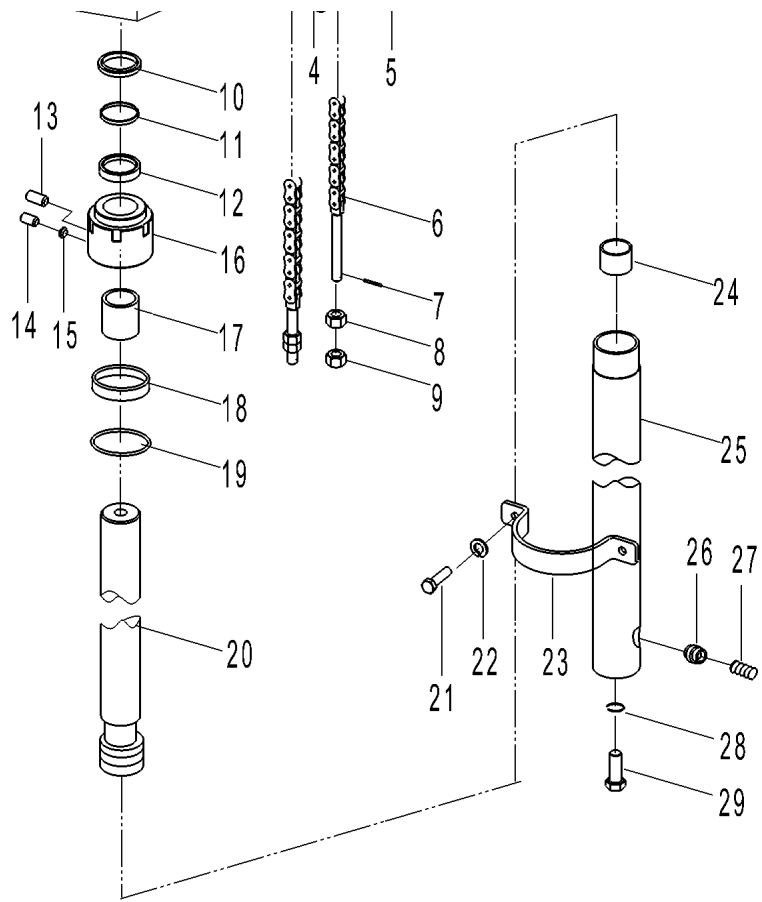
图55/FIG. 55 前起升油缸(三级全自由)/FRONT LIFT CYLINDER(FULL FREE 3-STAGE MAST)
