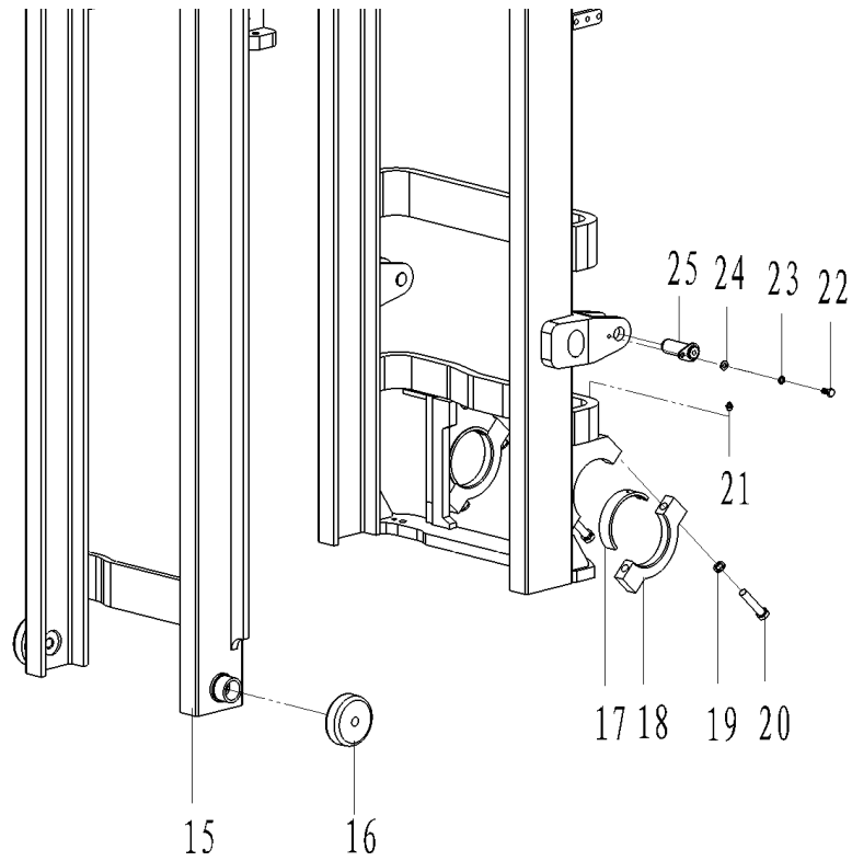
门架(基本型) / MAST(NORMAL MAST)
